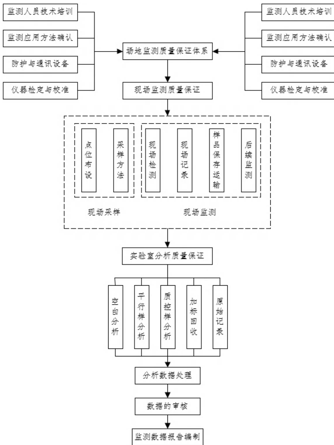
图 7.3-1 地块土壤污染状况调查采样与实验室检测分析质量保证体系框架图
